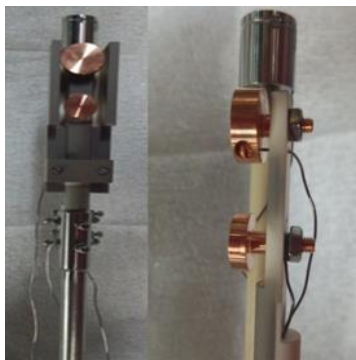
図1:現在使用しているカロリメータ
