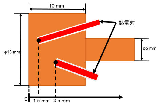
図2:新たに作成したカロリメータの模式図
