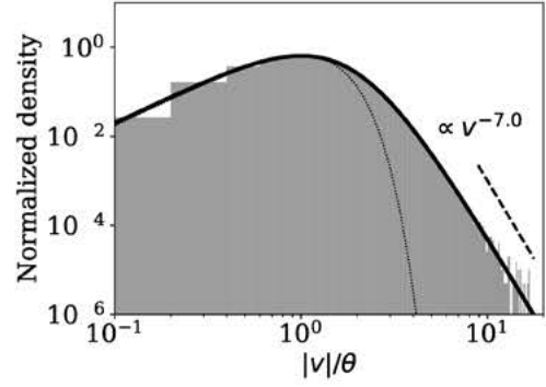
図 2 \kappa = 3.5 のカップ分布に従って乱数生成した粒子速度分布 (ヒストグラム) と解析解 (黒線). 黒の点線は内接マクスウェル分布.
