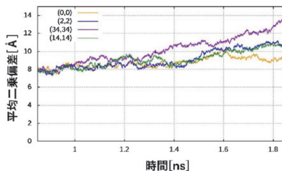
図15 共有結合への影響を調べるモデルでの平均二乗偏差の時間発展。傷の組数を、(0,0)、(2,2)、(14,14)、(34,34)の4つの場合について調べた。
