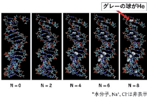
図9 水素結合に及ぼすトリチウム壊変効果の影響を調べるためのテロメアの初期構造。水素がヘリウムに壊変したグアニンの個数を N とする。 2N 個の水素原子がヘリウム3原子(グレーの球)に置き換えられる構造を初期状態として時間発展を、CHARMM36ポテンシャルを用いたNAMDコードでシミュレートする。
