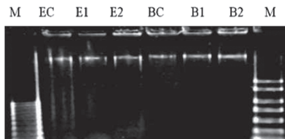
図9 イオン照射後の抽出 DNA の電気泳動結果。 略語：M-分子量マーカー、ECとBCはそれぞれEnterococcusとBacillusのPCI未照射のDNA ・E1、B1はそれぞれ2時間PCI照射後のDNA ・E2、B2はそれぞれ8時間PCI照射後のDNA
