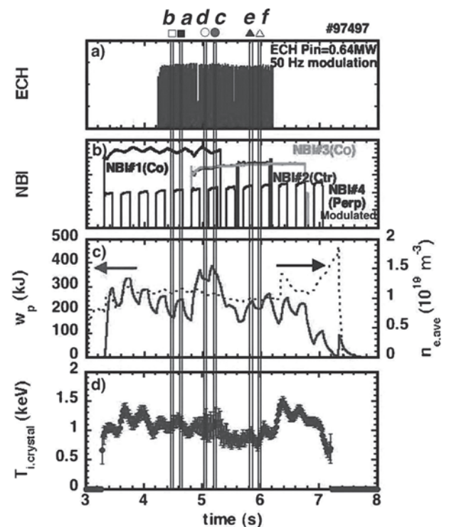
図5 CTS計測を行ったショットの代表的な放電波形。(a)CTSプローブビームの入射波形50 Hzで電力の100%矩形変調がかけられている。(b)接線 Co-NBI(#1, #3), Ctr-NBI(#2) および垂直 NBI(#4) (c)蓄積エネルギーと平均電子密度 (d)結晶分光のドップラー広がりから求めたイオン温度[12]。
