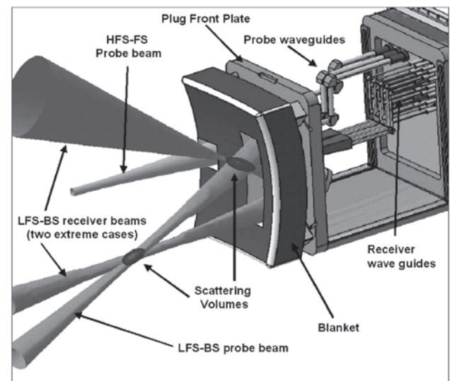
図8 ITER低磁場側CTS用受信アンテナと二つのプローブビーム入射アンテナおよびそれらのための開口部と導波管[15]。
