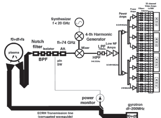
図4 LHDで用いられたCTS受信器のブロック図、主なコンポーネントは ノッチフィルター、ピンスイッチ、シンセサイザーで励振した4倍高調波発振器を局所発振器とするミキサー、中間周波増幅器と32チャンネルフィルターバンク、検波器および、ビデオアンプ等である[12]。
