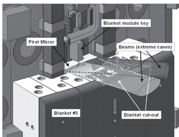
図9 プラズマ側から見たITER高磁場側CTS用受信ビーム（振り角の両極端を示してある）とそのためのブランケット開口部、プローブビームは低磁場側から入射されることを想定している（図8のHFS-FS Probe beam）[15]。
