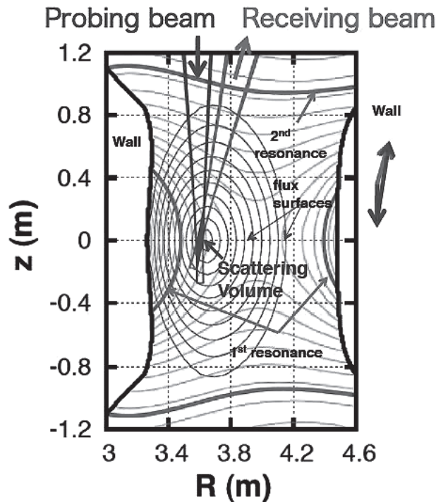
図6 LHDで行われたCTS計測のプローブ、受信ビーム(77GHz)の配置とLHDの磁場強度を2.4 Tに設定した場合の共鳴層の関係[12]。
