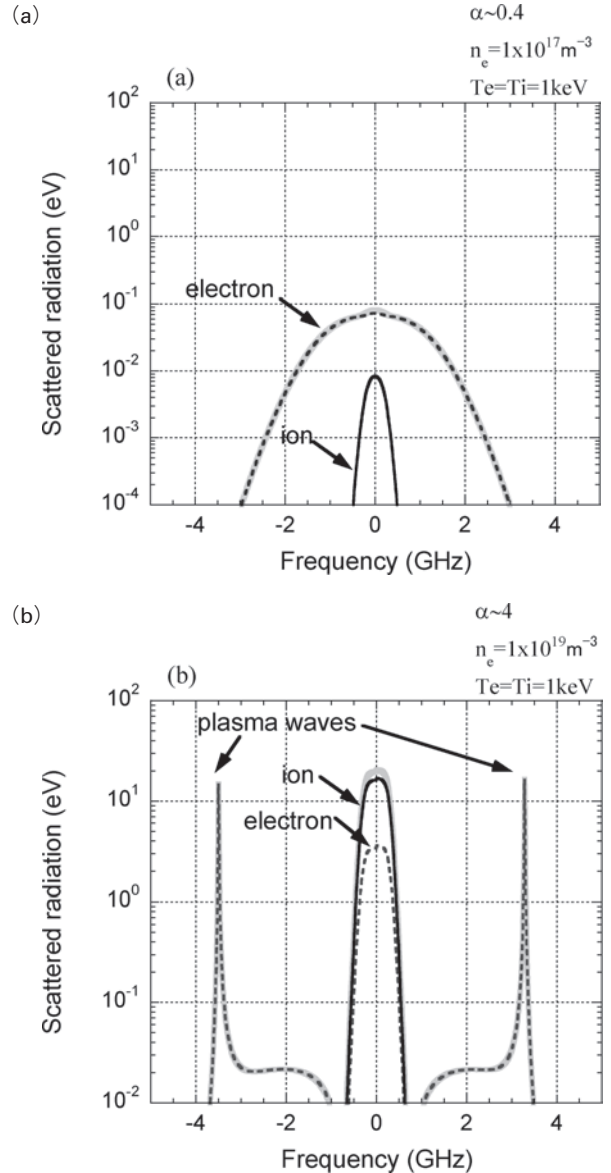
図3 サルピータパラメータによる CTS スペクトルの変化。 (a) \alpha = 0.4 , (b) \alpha = 4.0 .
