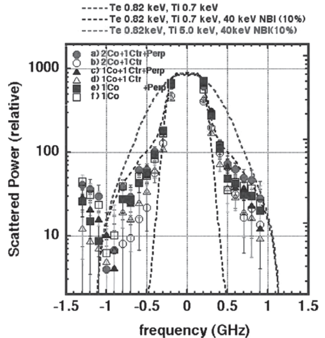
図7 図5のa-fで示された各時間でのCTSスペクトル。a) Co-NBI 2本 Ctr-NBI 1本、垂直NBI 重畳、b) Co-NBI 2本 Ctr-NBI 1本、垂直NBI 重畳なし、c) Co-, Ctr 各1本、垂直NBI 重畳、d) Co-, Ctr 各1本、垂直NBI 重畳なし e) Co 1本 垂直NBI 重畳、f) Co 1本 垂直NBI 重畳なしの各場合。測定された電子温度を0.82 keVを使って、イオン温度を0.7 keVとした場合と5 keVとした場合の垂直NBI有無の計算されたスペクトルが描かれている[12]。
