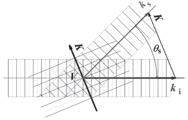
図1 入射波、電子密度揺動、散乱波の関係とそれらに対応した波数ベクトル \mathbf{k}_i 、 \mathbf{k}_s 、 \mathbf{K} 。 \theta_s は散乱角を示している。
