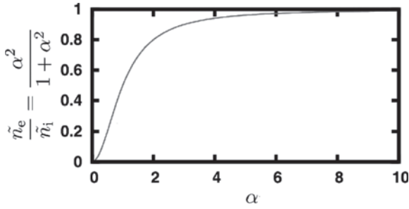
図2 サルピータパラメータ \alpha に対するイオン密度揺動に起因する電子密度揺動の大きさ。
